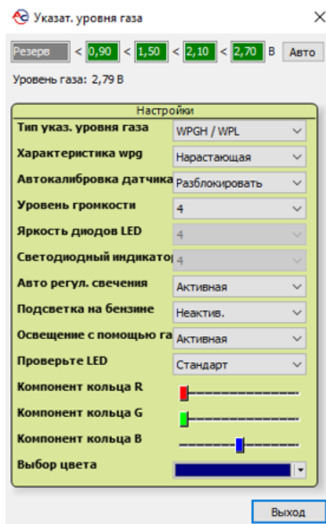
Рисунок 15 Окно конфигурации показателя уровня газа
