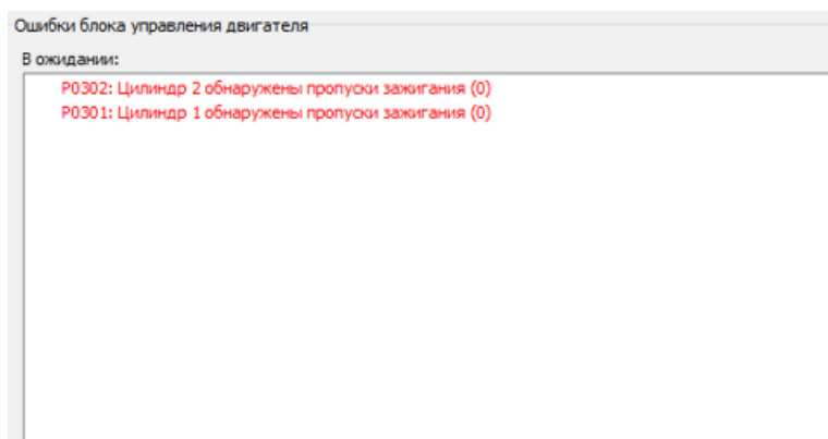
Рисунок 20 ОБД Вид закладки «Ошибки». Ошибки ОБД
