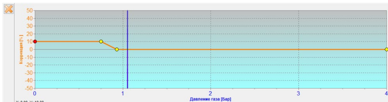
Рисунок 28 Карта «Коррекция давления газа»
