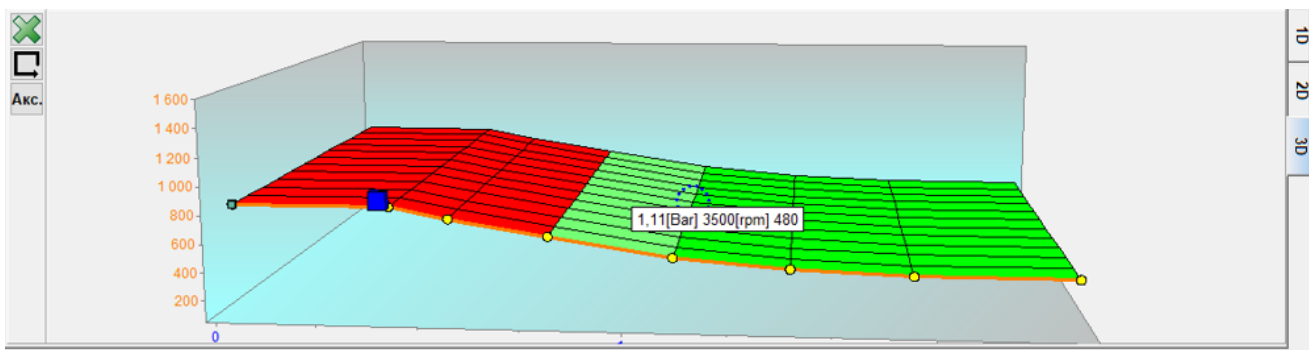
Рисунок 24 Карта множителей 3D
