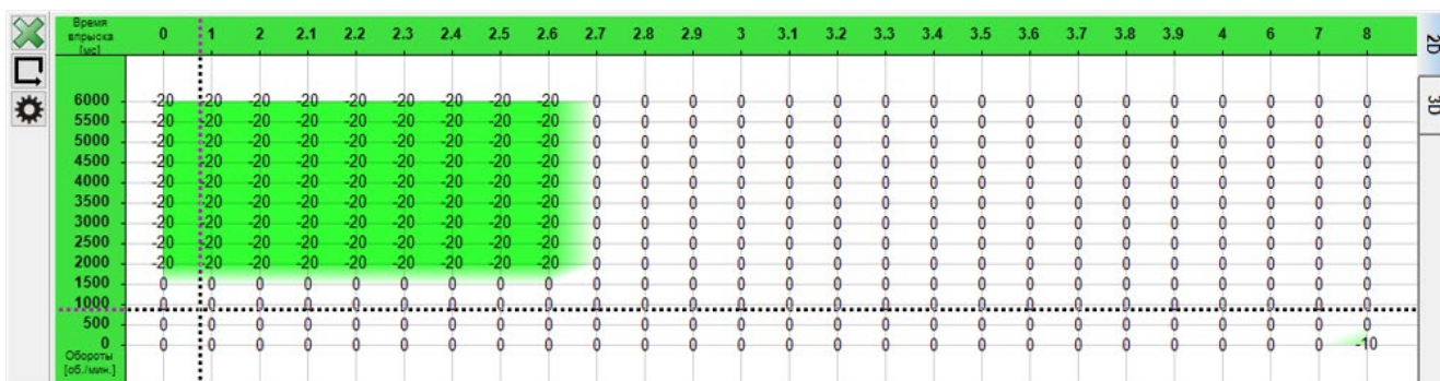
Рисунок 25 Вид карты коррекции оборотов
