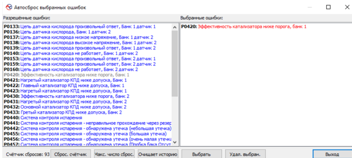
Рисунок 21 Вид конфигурации автоматического удаления неисправностей ОБД
