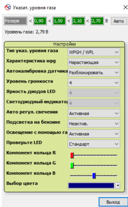
Рисунок 40 Окно конфигурации LED-600
