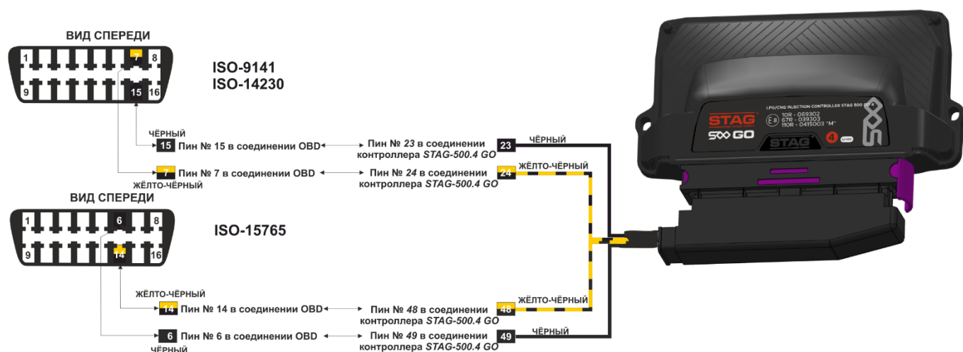
Рисунок 4 Конфигурация жгута контроллера диагностических протоколов CAN (ISO-15765) и
