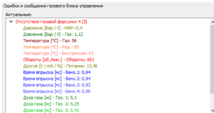
Рисунок 19 «Замороженная рамка» ошибки форсунки
