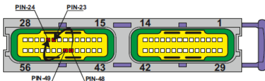
Рисунок 5 Изменение соединения в разъеме контроллера STAG 500 для диагностического протокола K-Line
