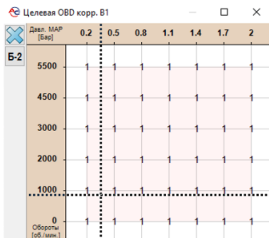
Рисунок 37 Карта целевых коррекций ОБД
