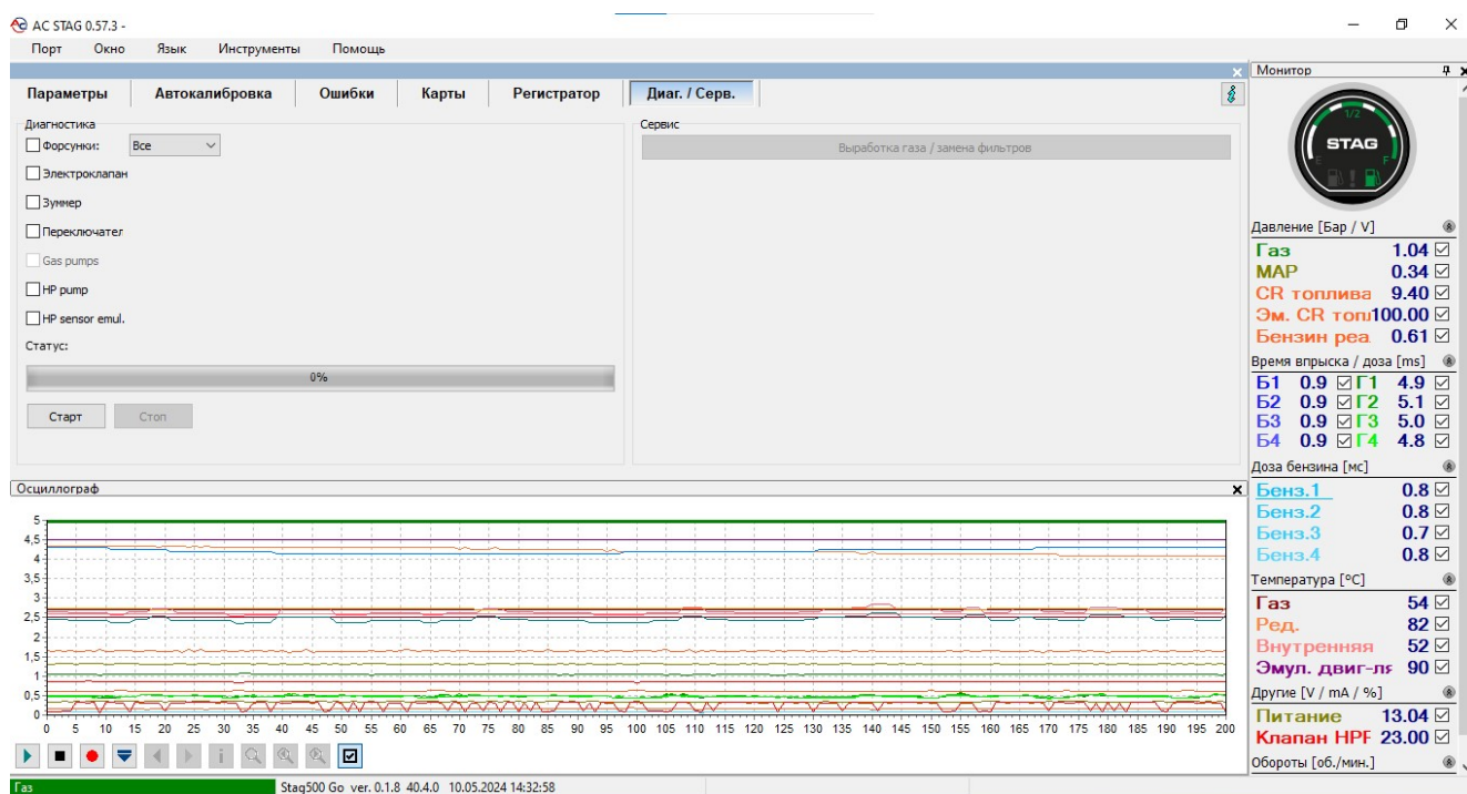
Рисунок 38 Окно «Диагностика и сервис»
