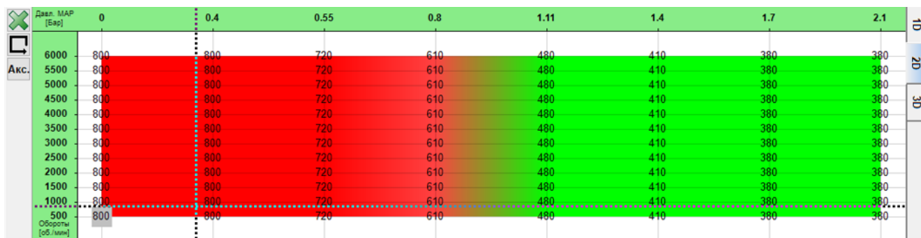
Рисунок 23 Карта множителей 2D
