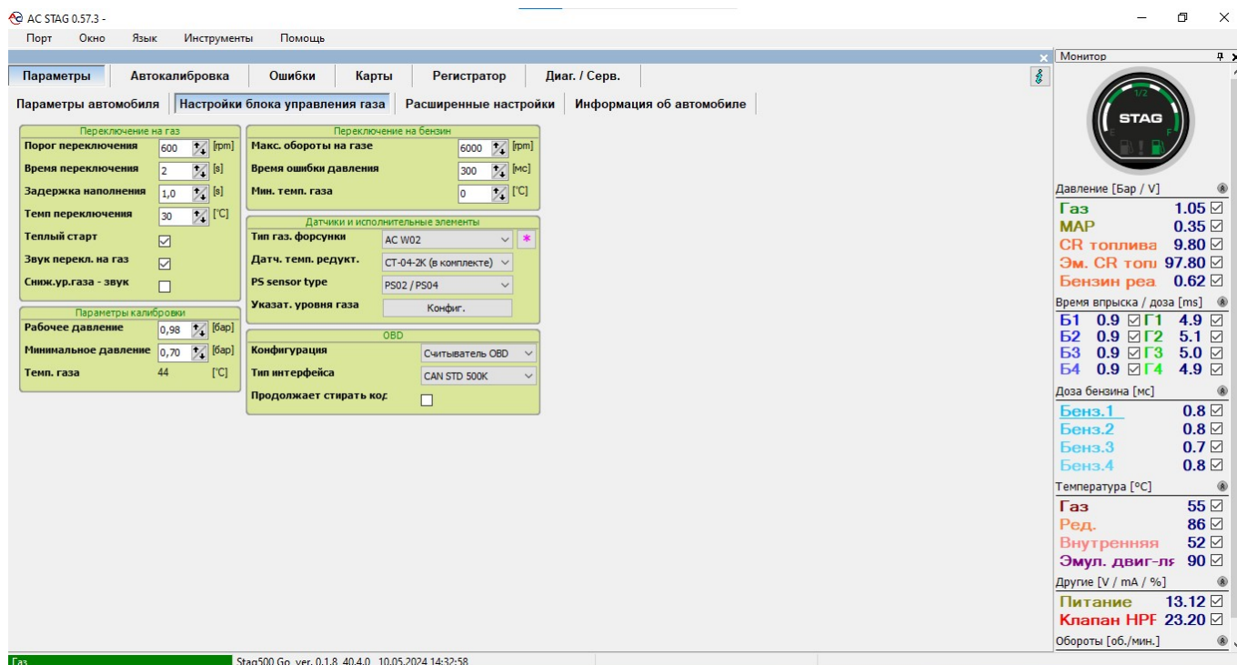
Рисунок 7 Окно «Параметры» (настройка контроллера газа)
