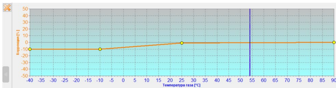
Рисунок 27 Карта «Коррекция температуры газа»
