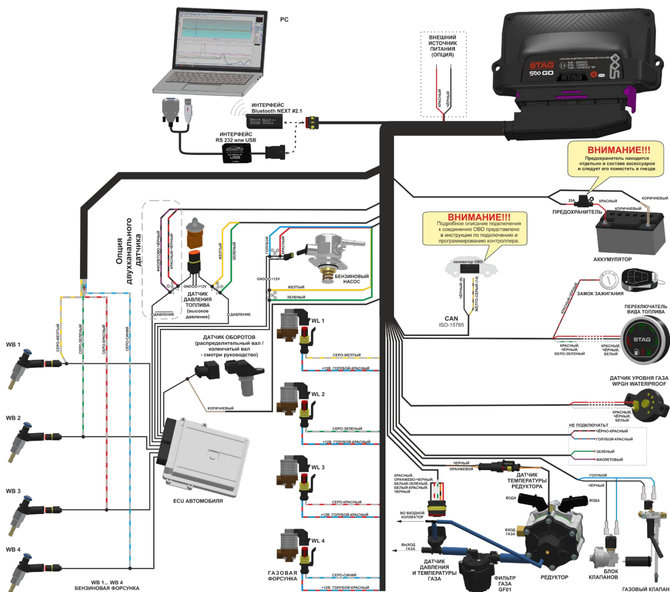
Рисунок 1 Схема подключения STAG 500 GO 4 к автомобильному оборудованию
